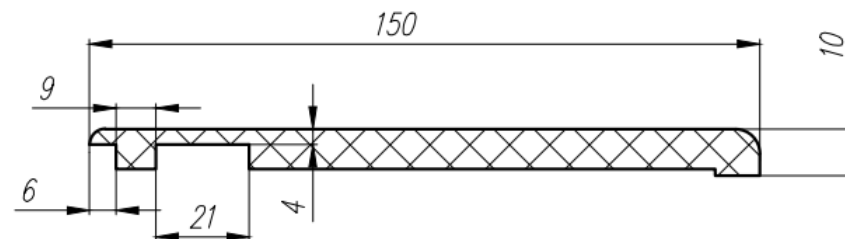
Q-наличник плоский 150x10
