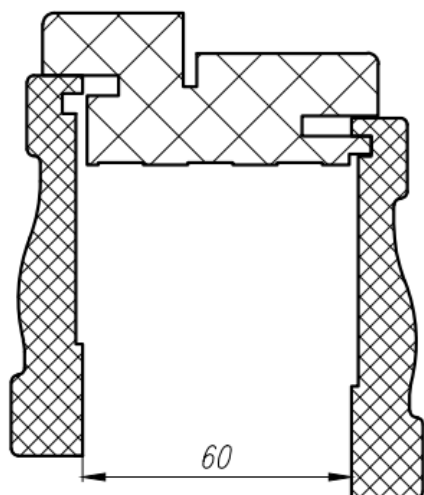
Стыковка без расширителя
