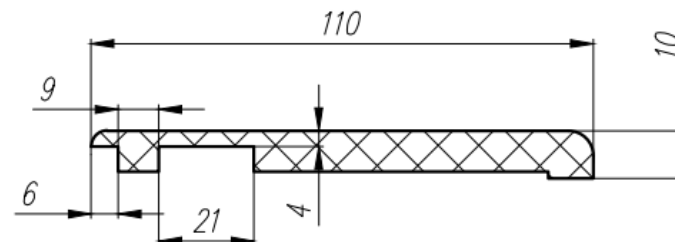
Q-наличник плоский 110x10
