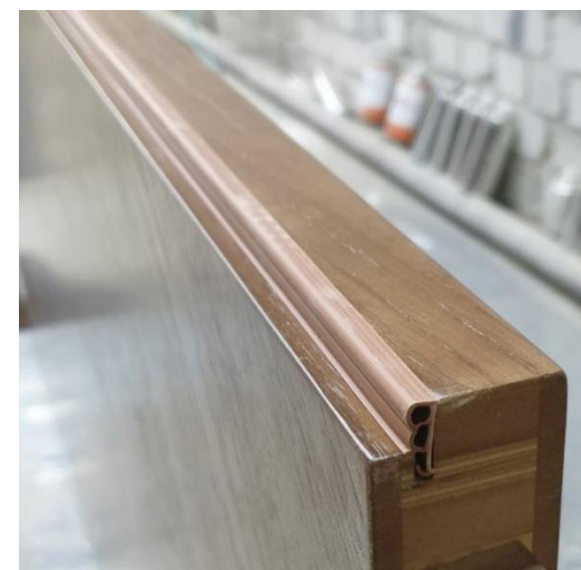
Торец RQ полотна в шпоне с уплотнителем
