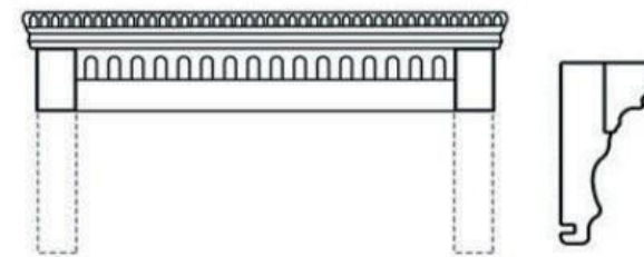
Карниз Россo с багетом Британия
