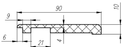
Q-наличник плоский 90x10
