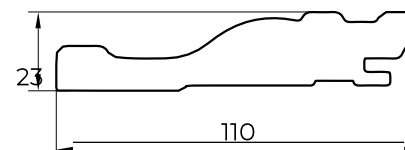
плинтус Модерн 1950(-20)x110x23 мм
